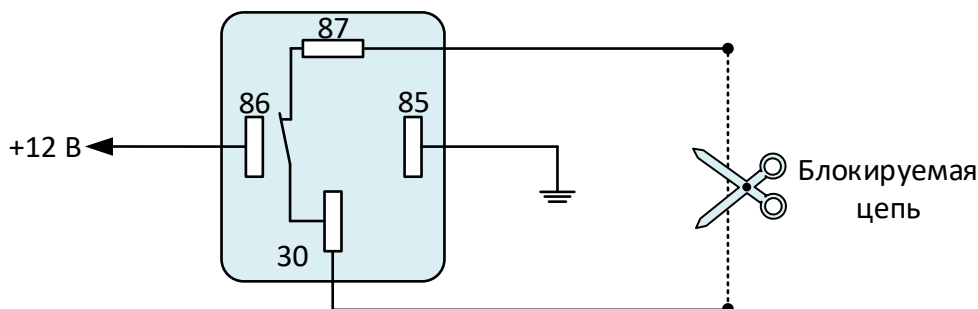
Рисунок Г.3 – Дистанционное блокирующее реле
