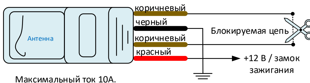
Рисунок Г.1 - Беспроводное радиореле
