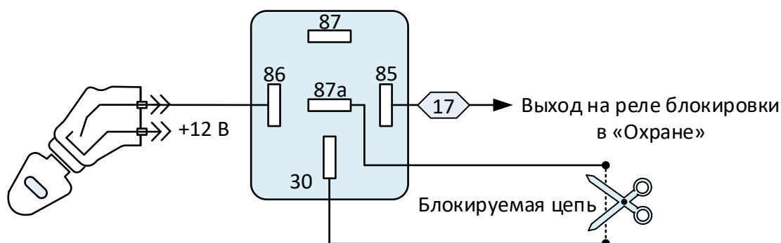
Рисунок Г.2 – Реле блокировки в охране
