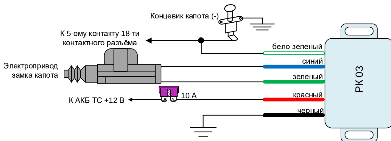
Г.4 – Схема подключения реле PK 03
